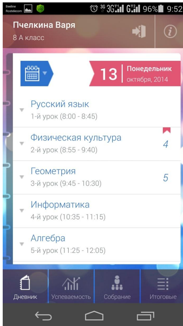
Рис. 2. Вкладка «Дневник»
