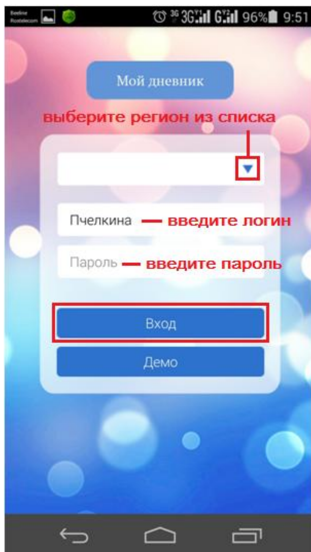
Рис. 1. Окно авторизации
